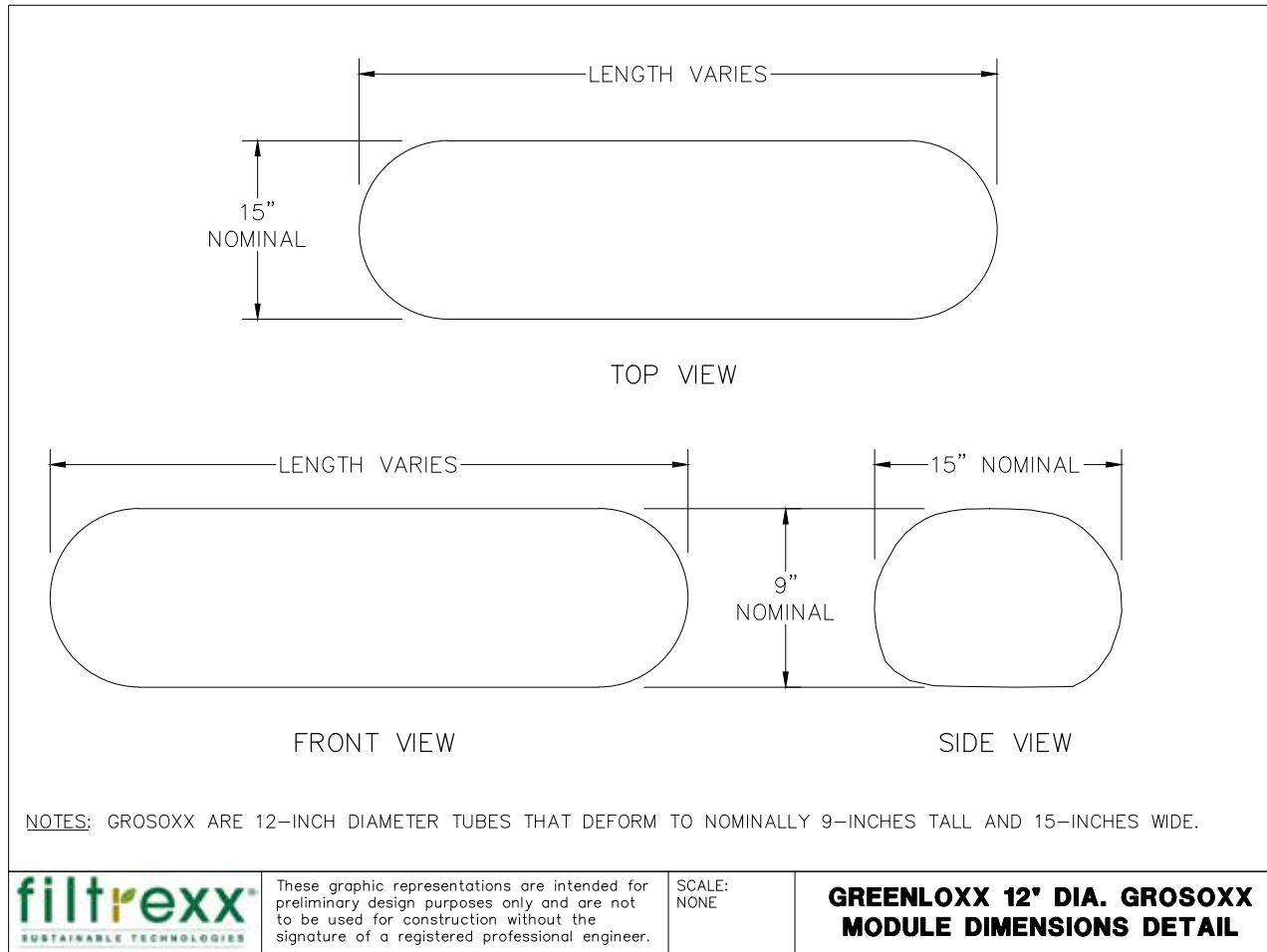
Figure 2.2. Filtrexx® GreenLoxx® 12" GroSoxx® Module Dimensions Detail
