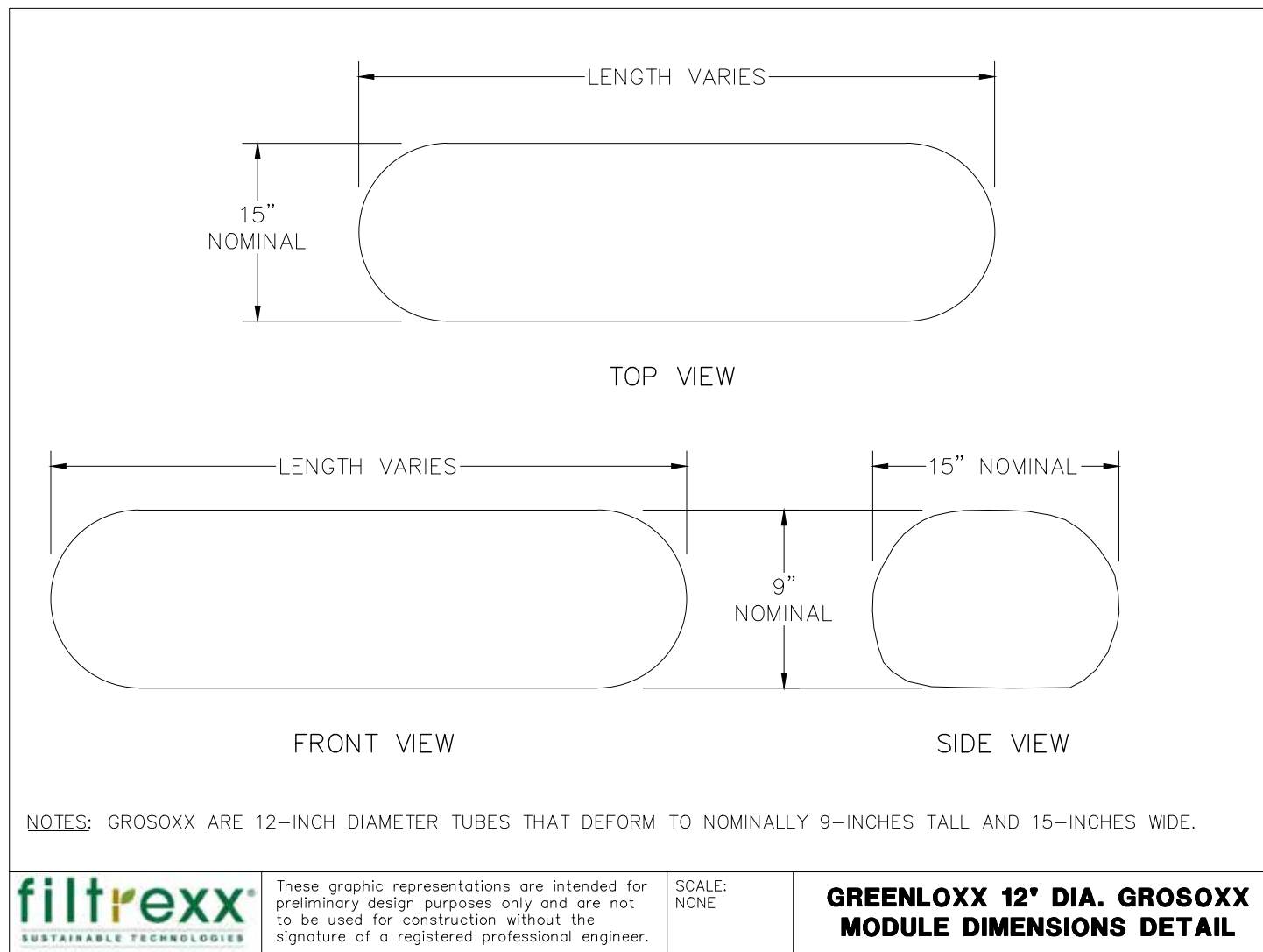
Figure 1.3. Filtrex® GreenLoxx® 12" GroSoxx® Module Dimensions Detail
